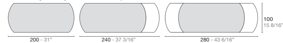
C/3098/S Larghezza tra gambe - Width between legs cm 91,5
