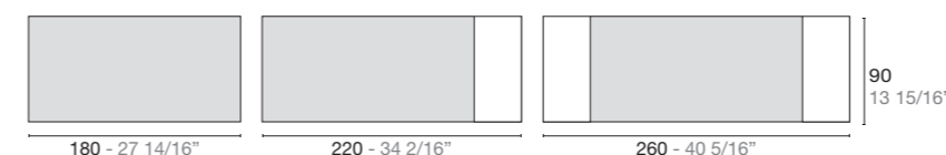
C/3100/S Larghezza tra gambe - Width between legs cm 134
