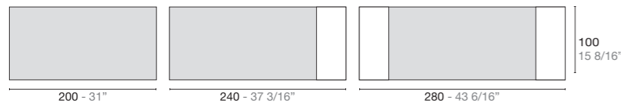
C/3157/L Larghezza tra gambe - Width between legs cm 154
